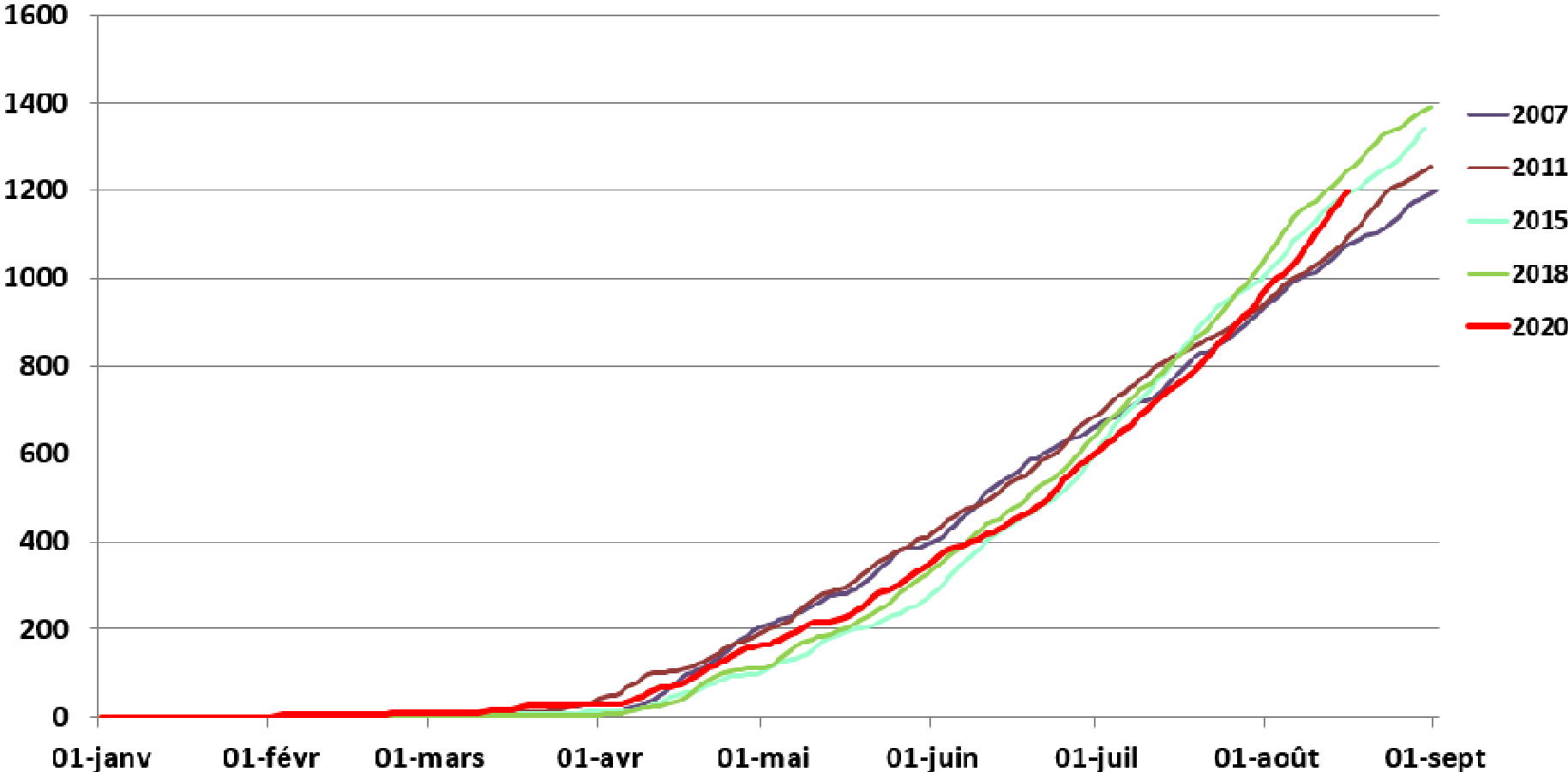
Somme des T°C en base 10 depuis le 1er janvier Millésimes précoces Météo France - Poste de Beaune
